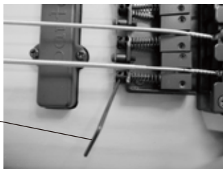
M3六角レンチ
